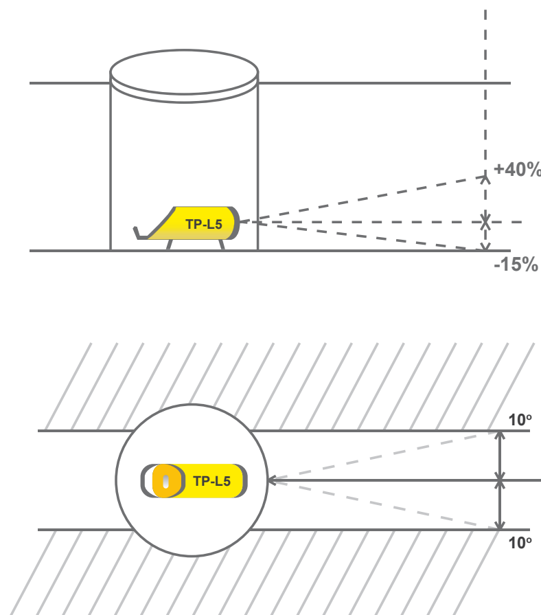
Rys.: Sposób wyznaczenia spadku (rys. górny) i kierunku (rys. dolny) za pomocą lasera liniowego wstawionego do studzienki kanalizacyjnej
